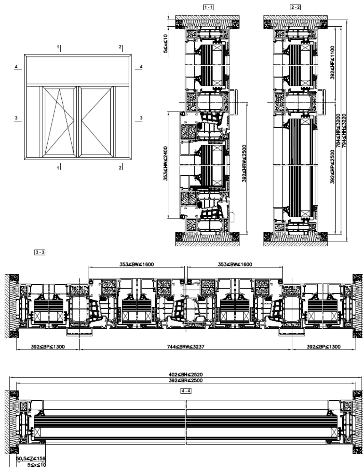
Rys.21. Zależności wymiarowe dla dwuskrzydłowego zestawu okiennego z doświetlami i nadświetłem MB - 86EI w klasie odporności ogniowej EI30 /EW30
