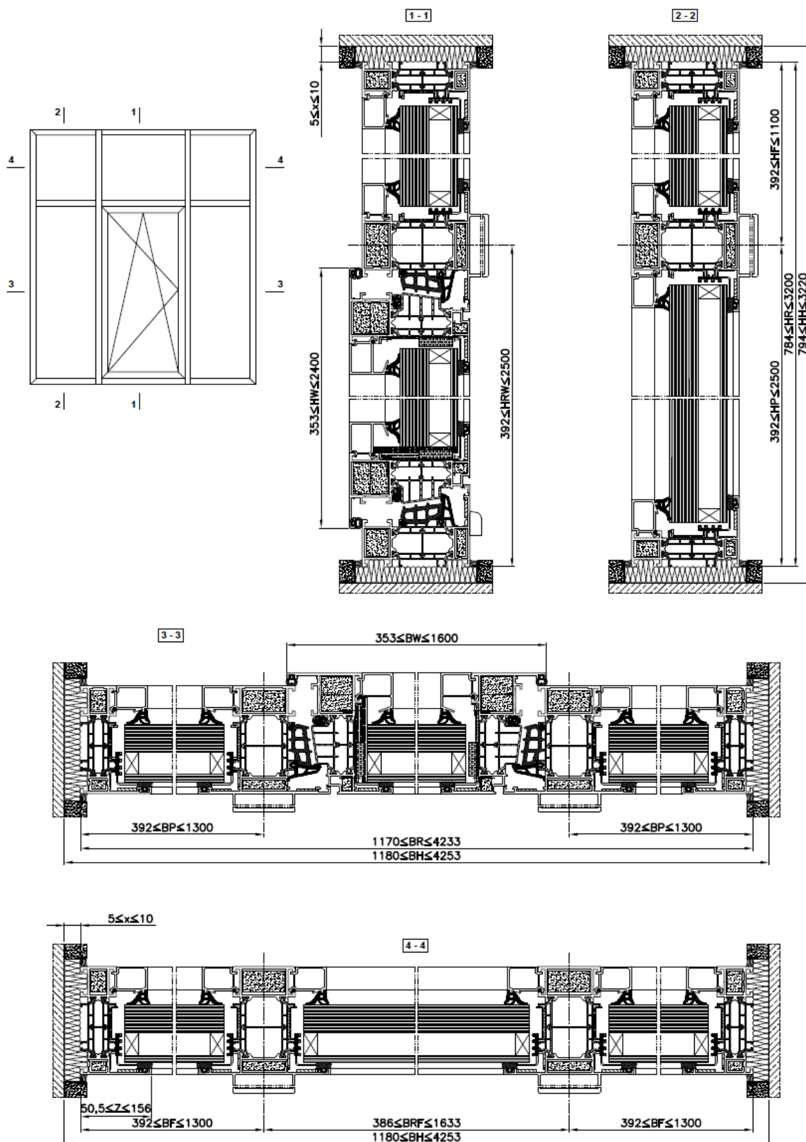
Rys.20. Zależności wymiarowe dla jednoskrzydłowego zestawu okiennego z doświetlami i nadświetlami MB - 86EI w klasie odporności ogniowej EI30 /EW30
