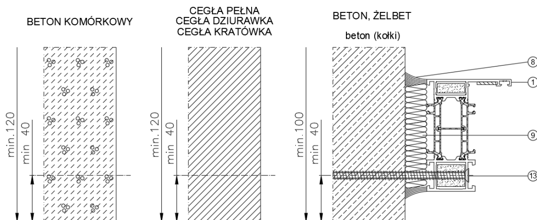
Rys.9. Schematy osadzania okien i zestawów okiennych MB - 86 EI w ścianach z różnych materiałów, z zastosowaniem wkrętów do betonu lub kołków rozporowych
