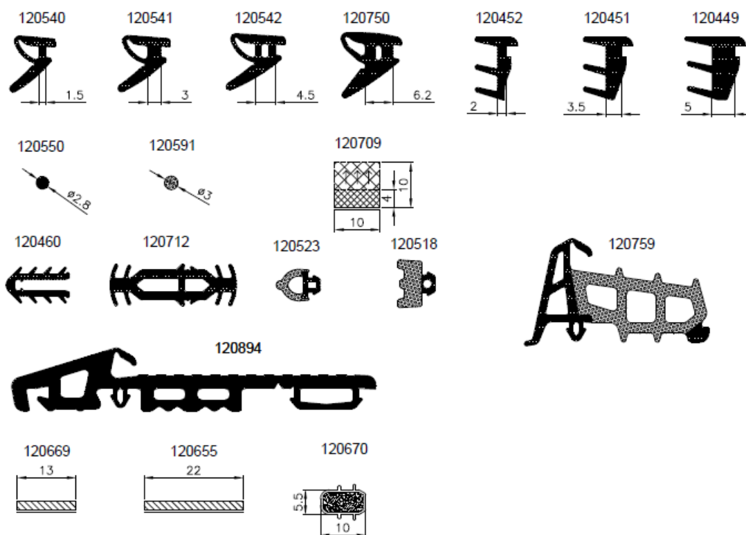
Rys.A8. Uszczelki, taśmy i uszczelki pęczniące
