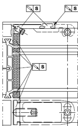
Rys.25. Połączenie typu „T” kształowników przewiązek ze stojakami ościeżnic i słupkami metodą kołkowania
