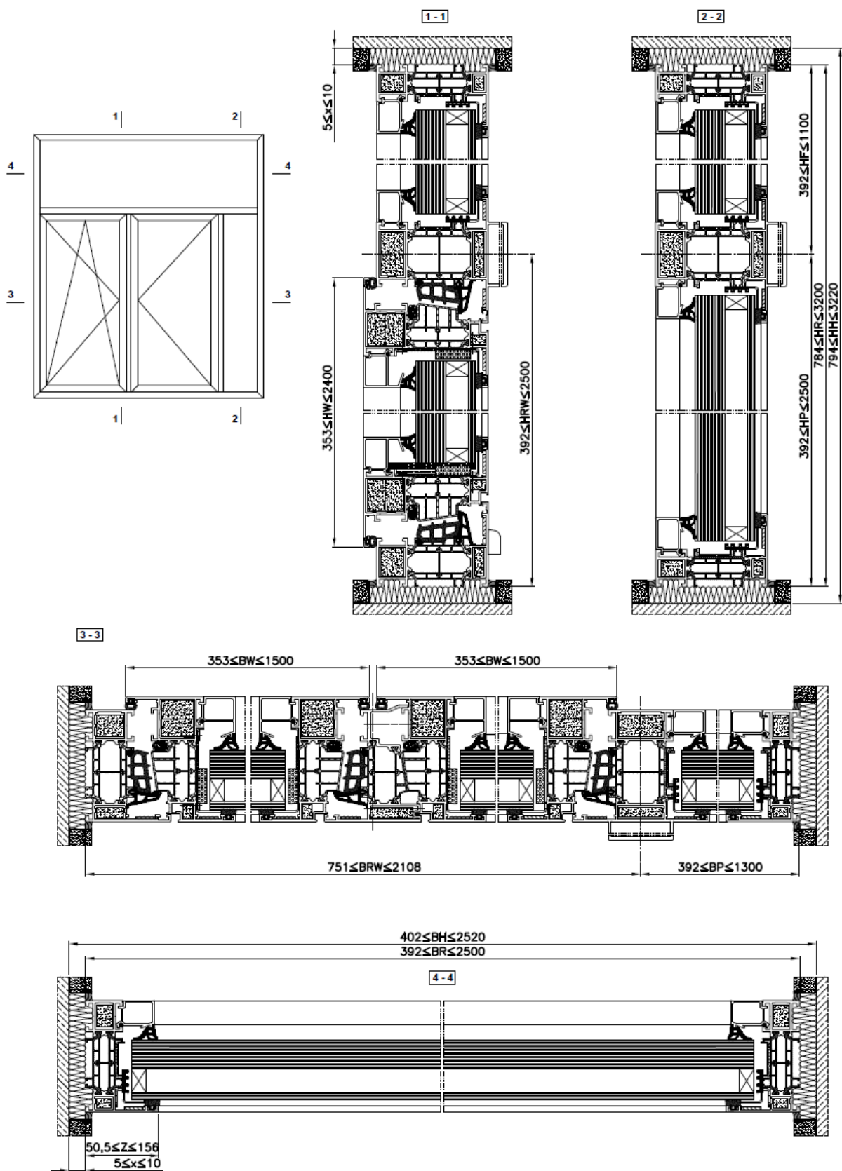
Rys.22. Zależności wymiarowe dla dwuskrzydłowego zestawu okiennego z doświetłem i nadświetłem MB - 86EI w klasie odporności ogniowej EI30 /EW30
