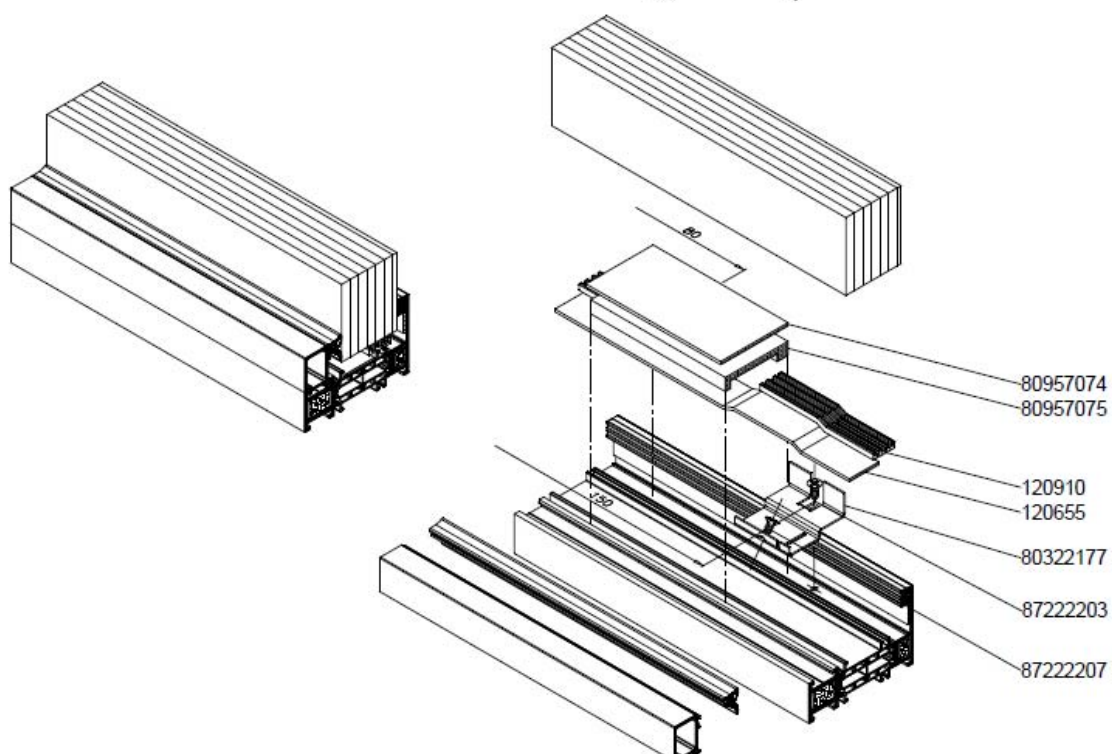
Rys.33. Elementy osadzenie wypełnień w skrzydle okiennym i w oknie stałym, doświetlu i nadświetlu
